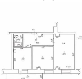
План квартиры
