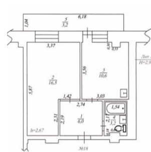
План квартиры
